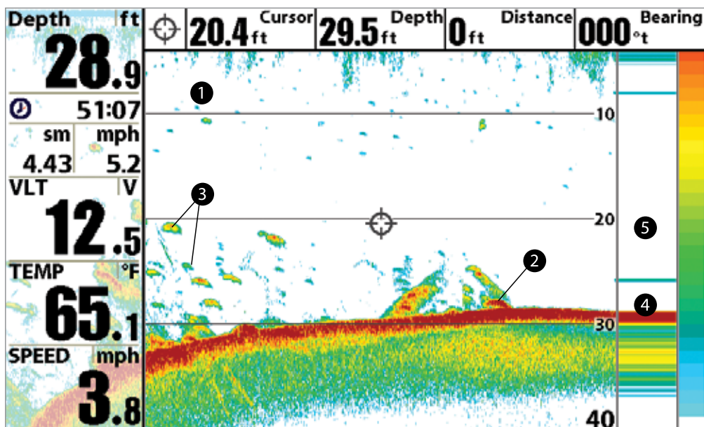
Обзор сонара: оригинальная палитра
